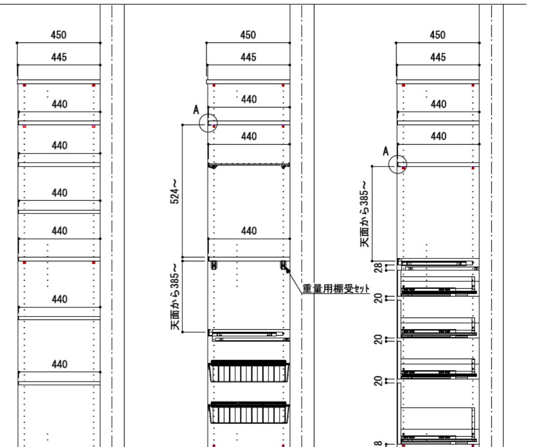
A-A' 断面
