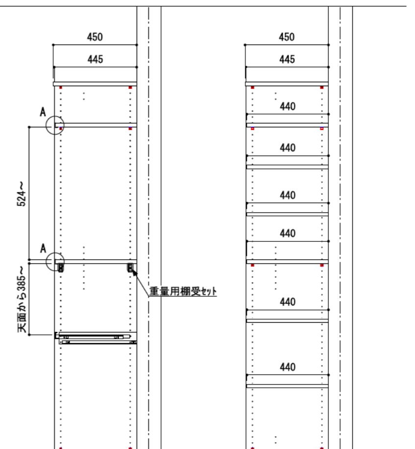
A-A' 断面
