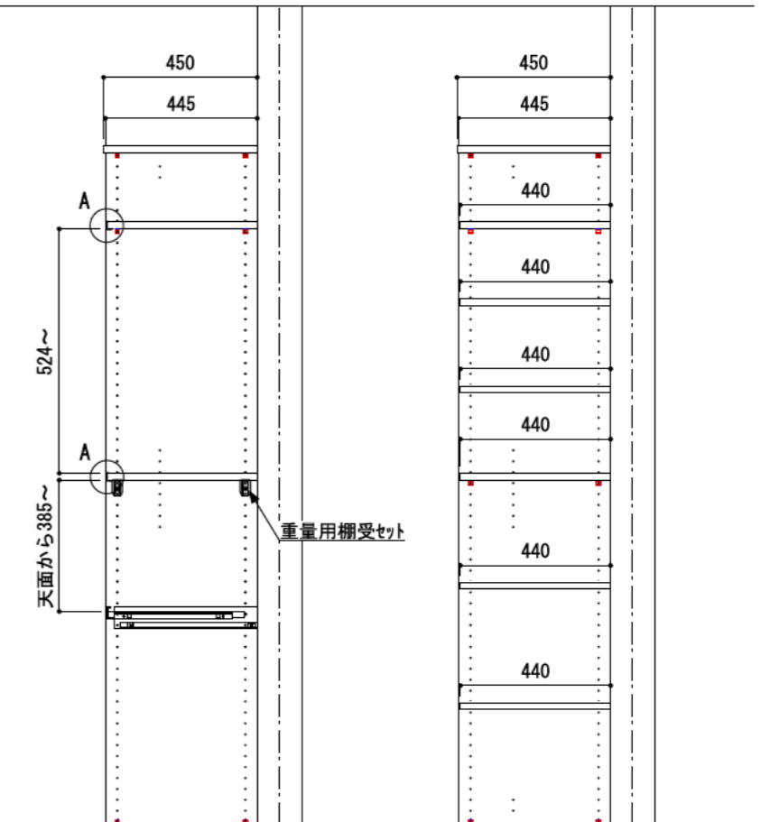
A-A' 断面
