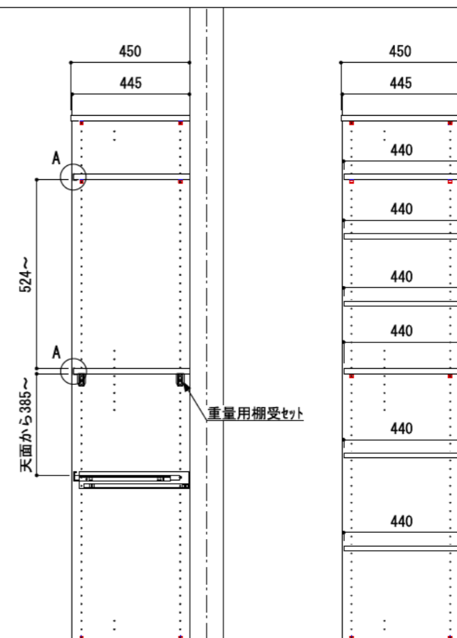
A-A' 断面
