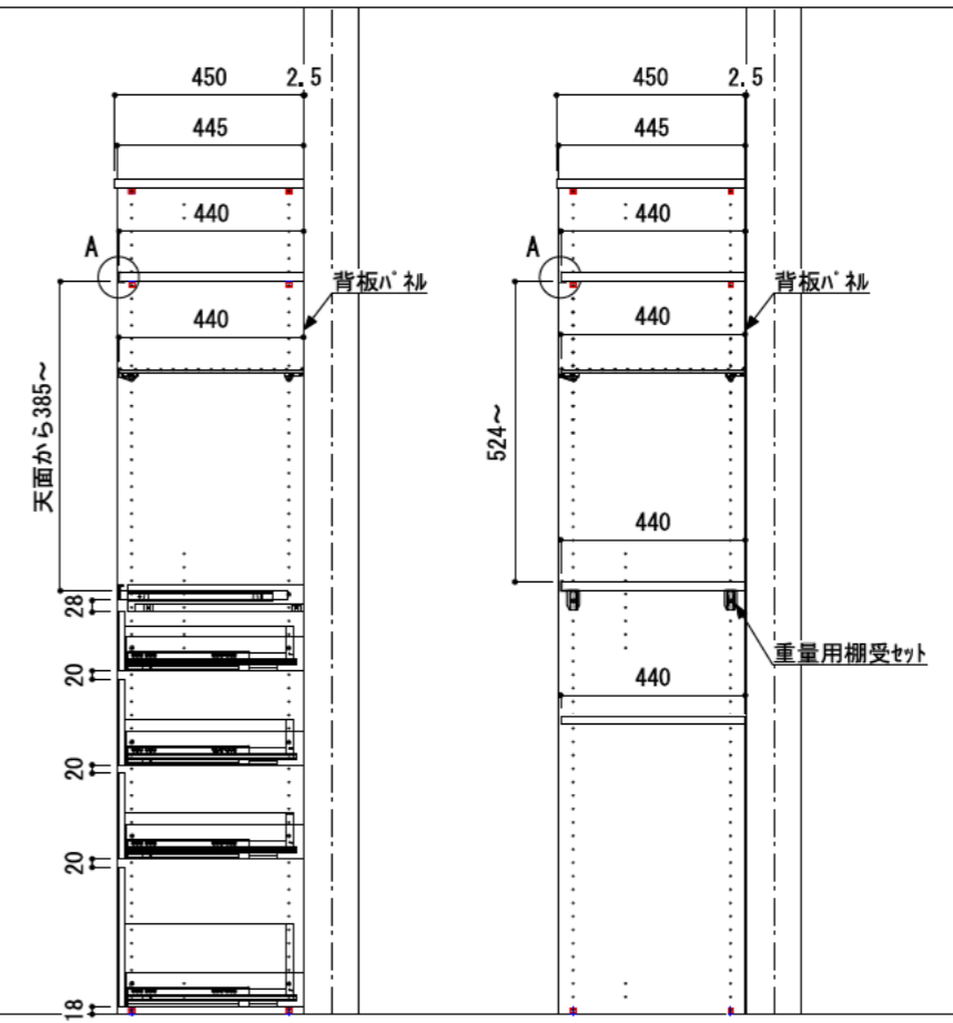
A-A' 断面
