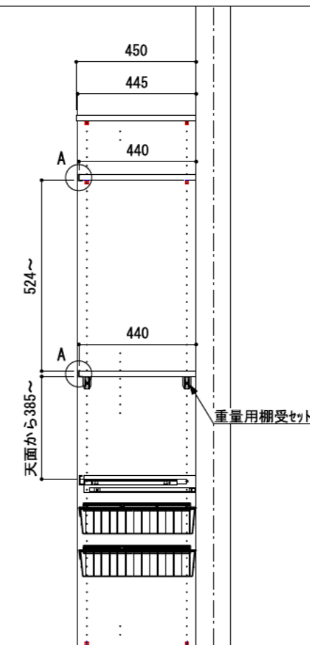
A-A' 断面
