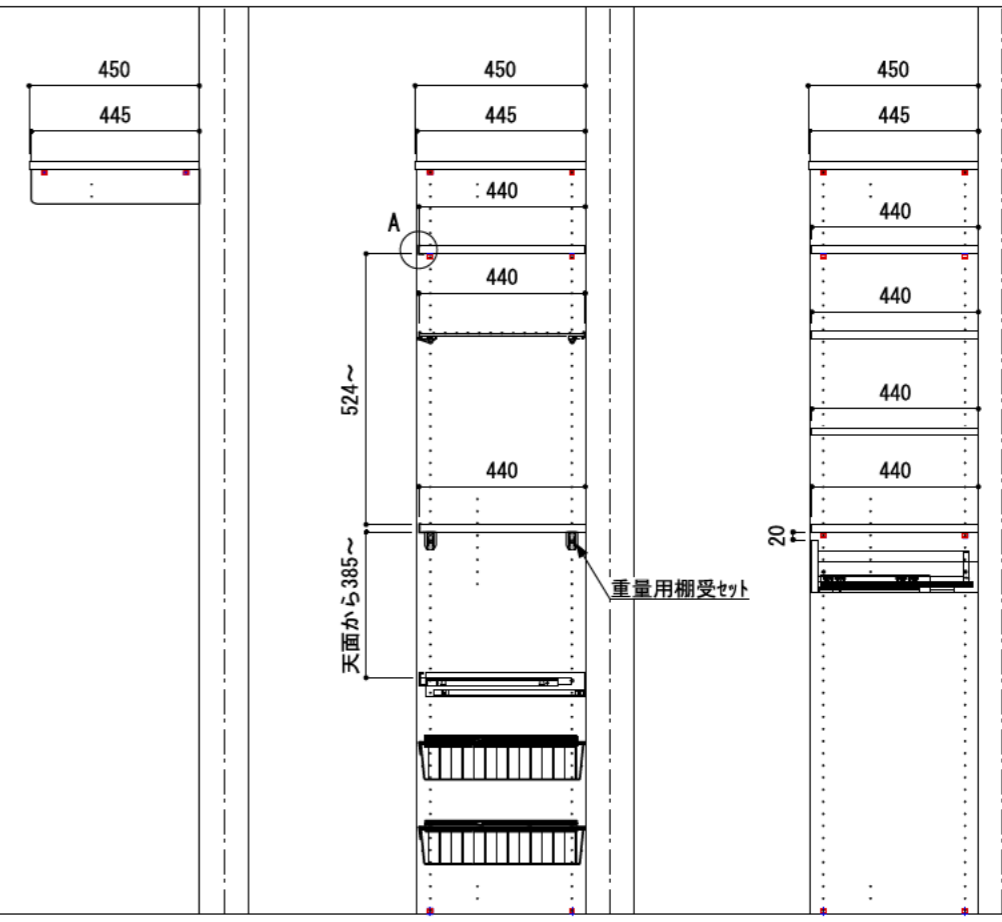
A-A' 断面
