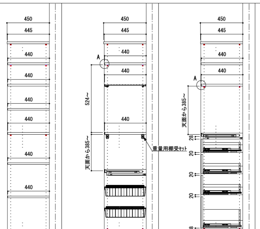
A-A' 断面
