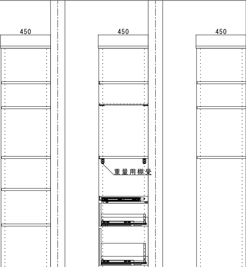
A-A' 断面
