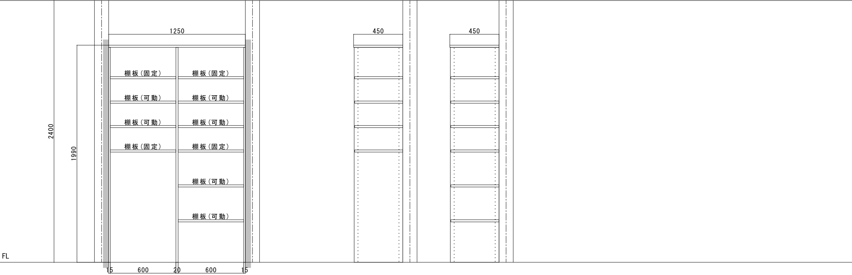
A-A' 断面
