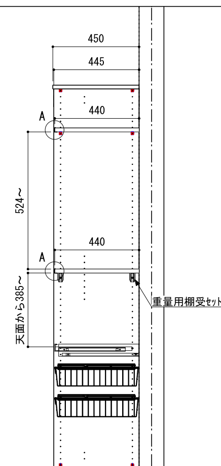
A-A' 断面
