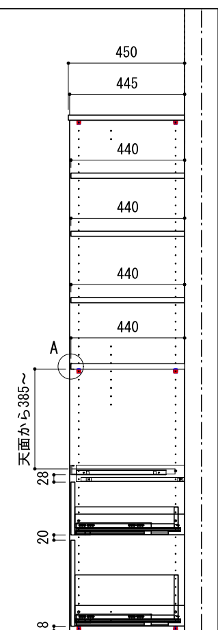
B-B' 断面
