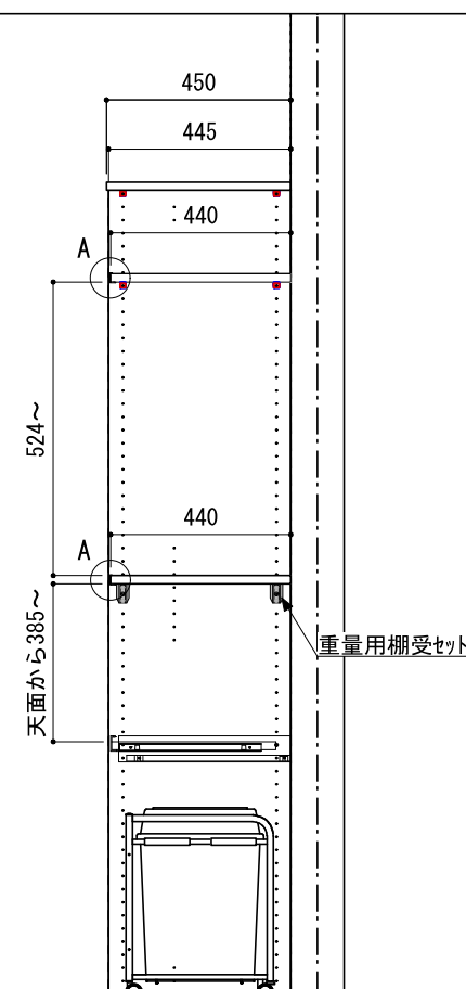
B-B' 断面
