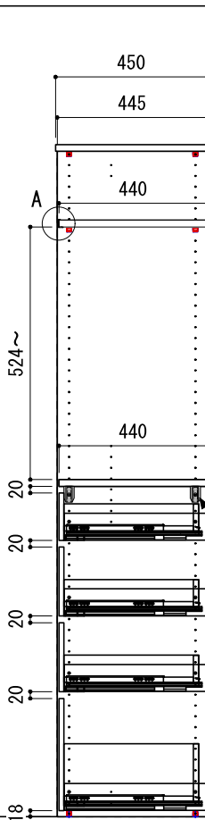
A-A' 断面
