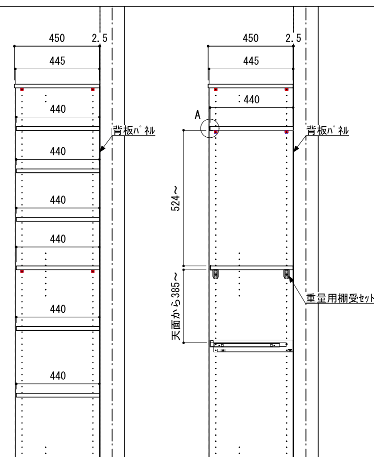
A-A' 断面
