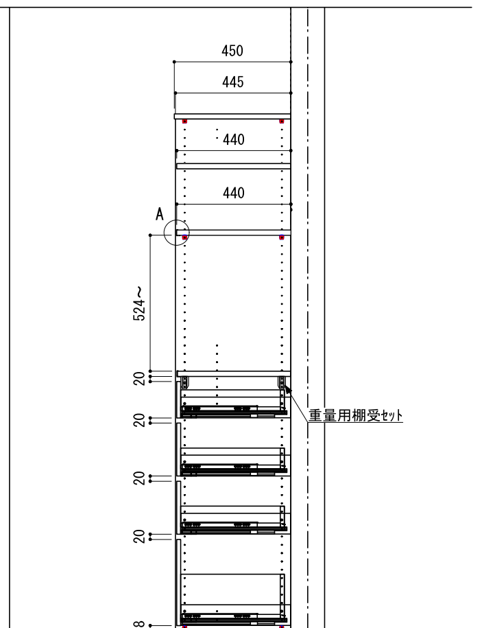
B-B' 断面
