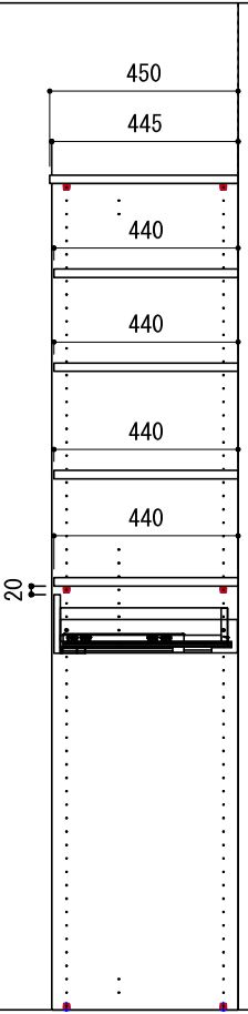
C-C' 断面
