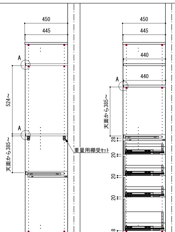
A-A' 断面
