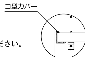
A-詳細図
