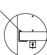
A-詳細図
