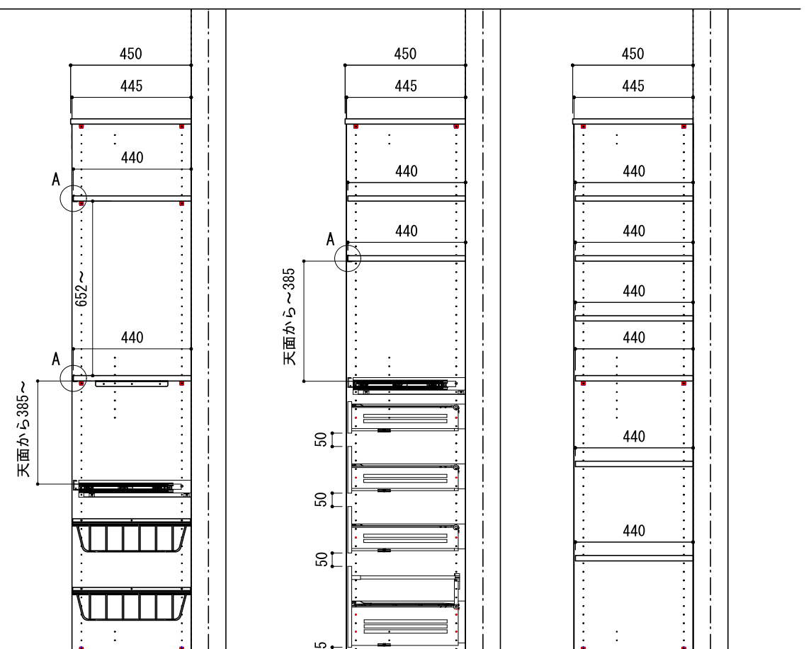
A-A' 断面
