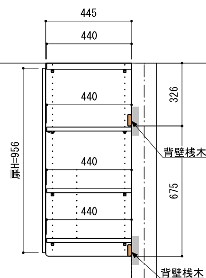
A-A' 断面
