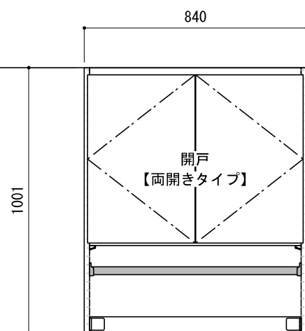
正面図（外観）
