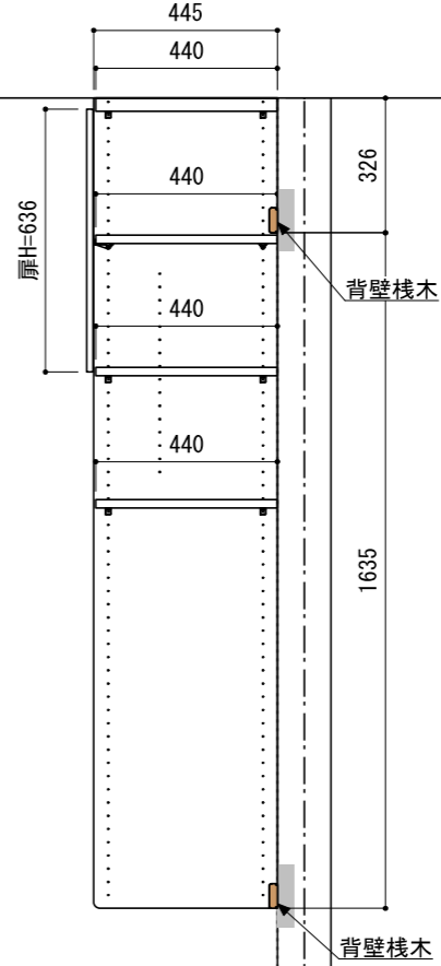
A-A' 断面
