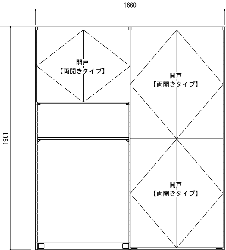
正面図（外観）
