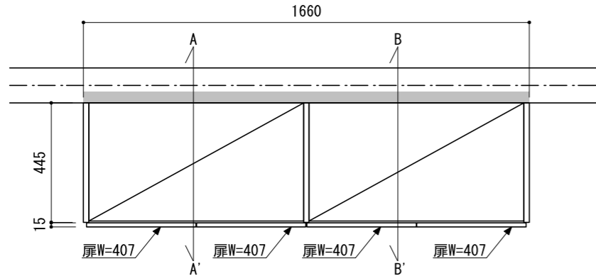
正面図（外観）
