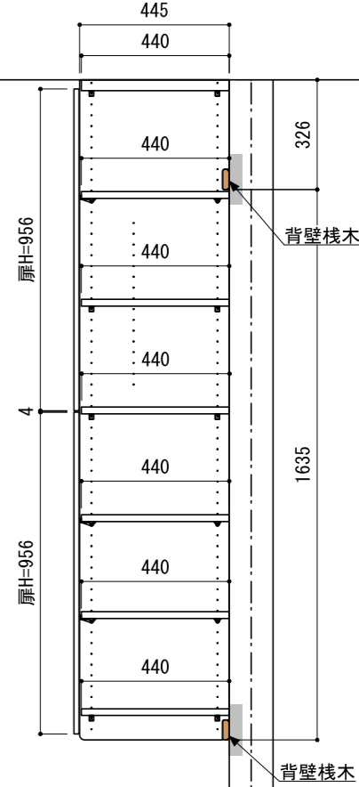
B-B' 断面
