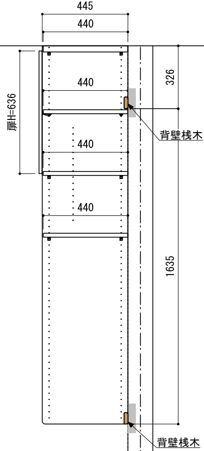
A-A' 断面
