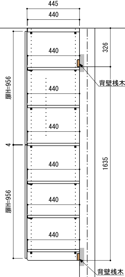
B-B' 断面
