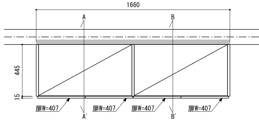
正面図（外観）
