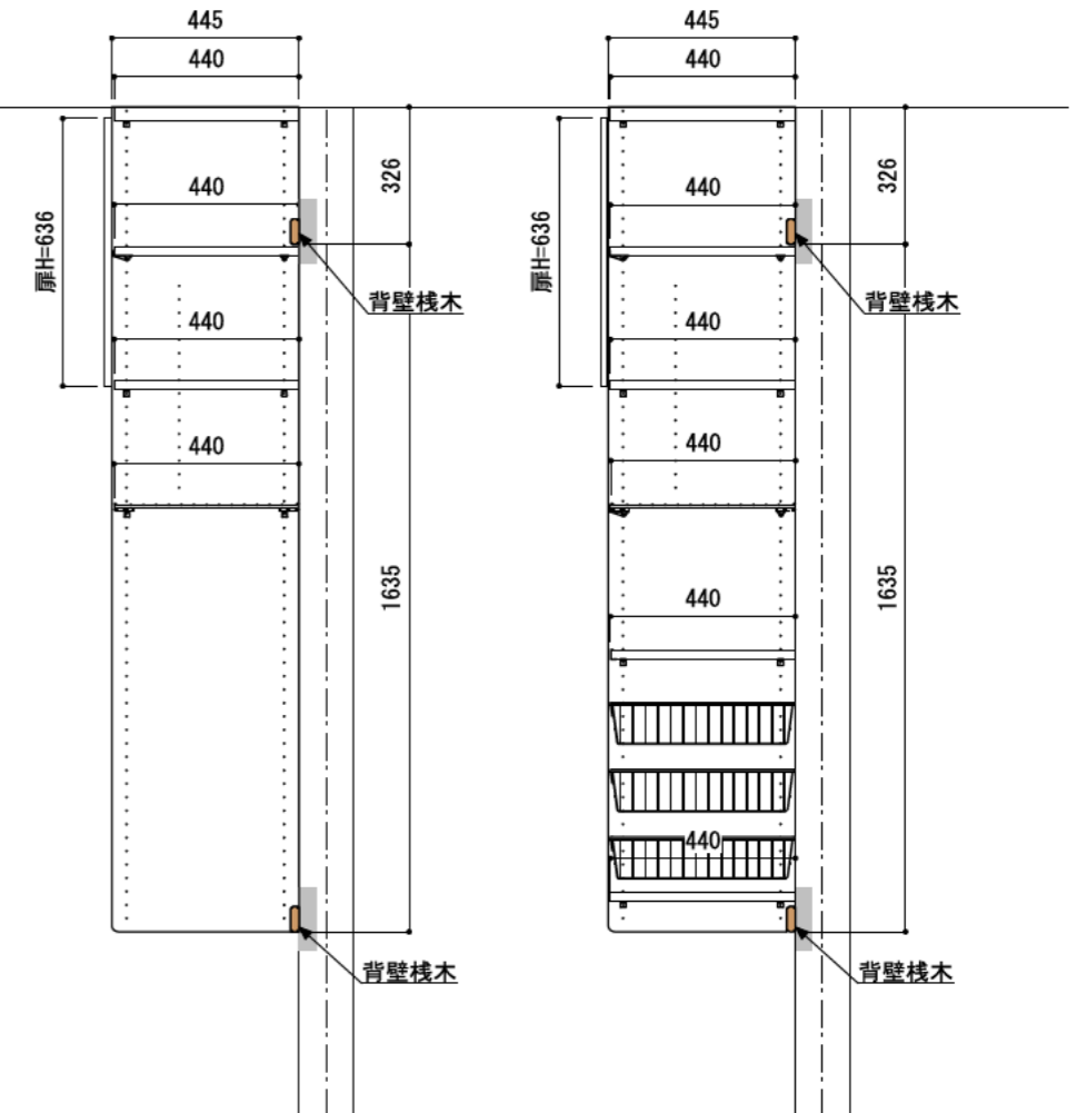
A-A' 断面
