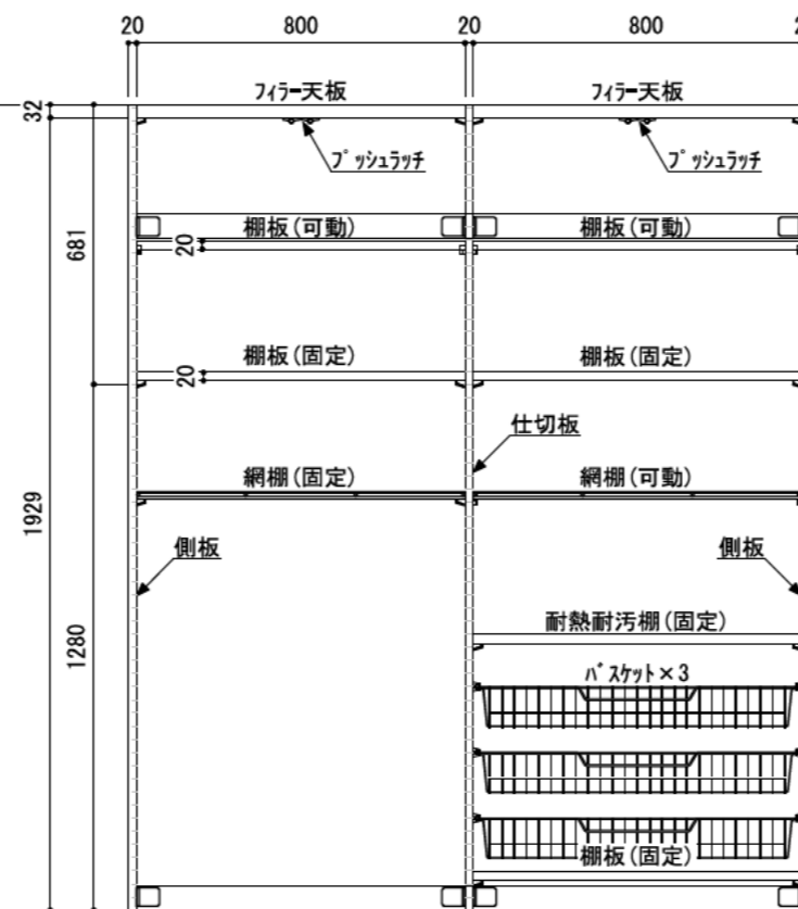
正面図（扉内部）
