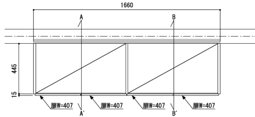
正面図（外観）
