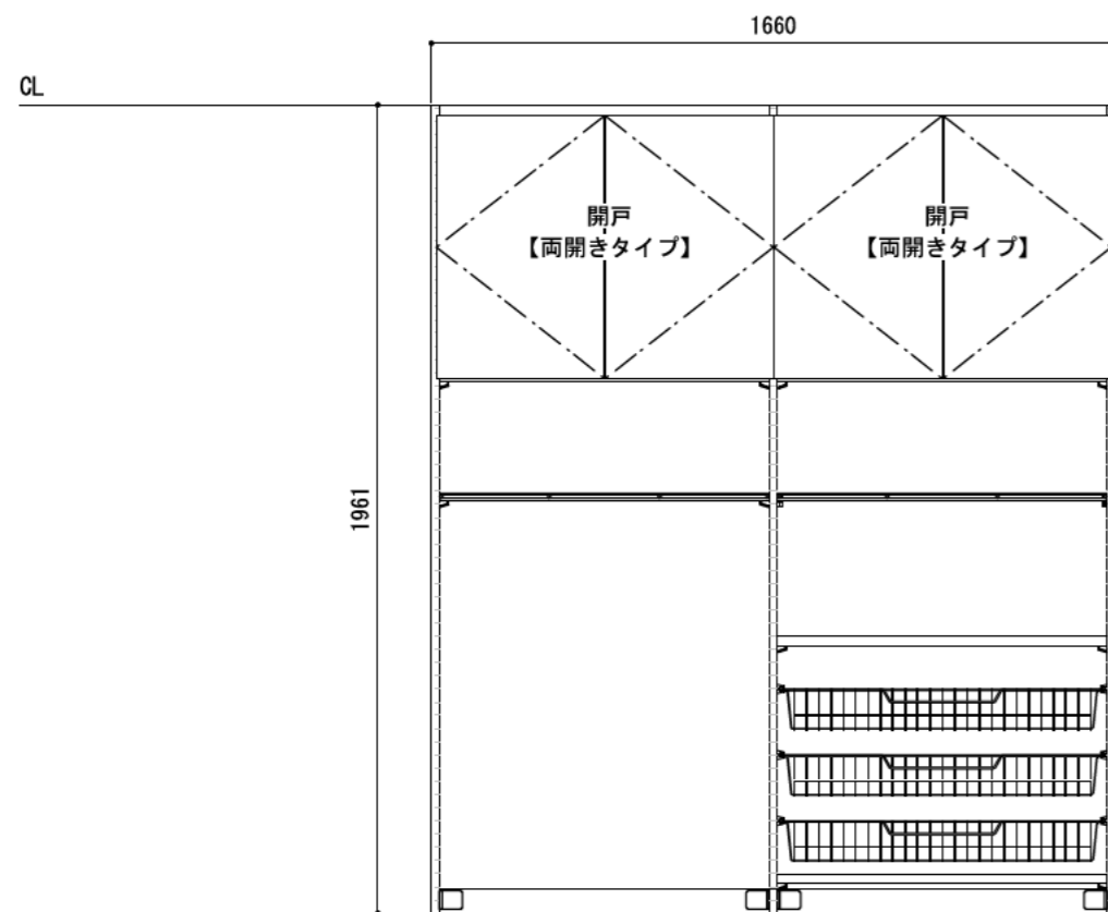
正面図（外観）
