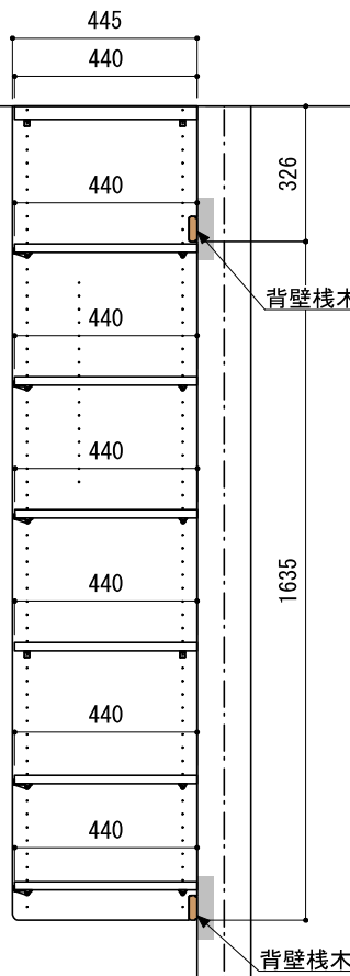
B-B' 断面
