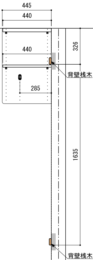
A-A' 断面
