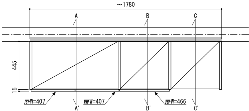
正面図（外観）
