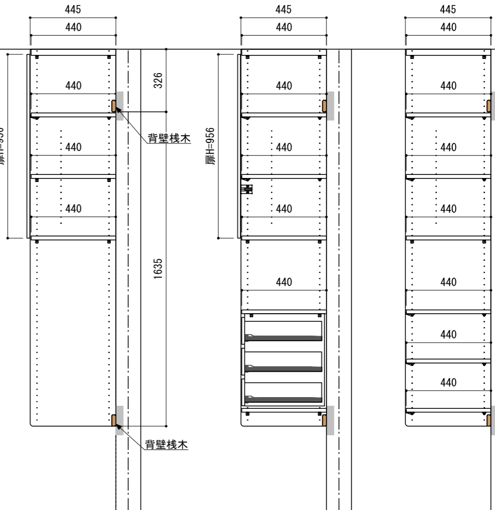
A-A' 断面
