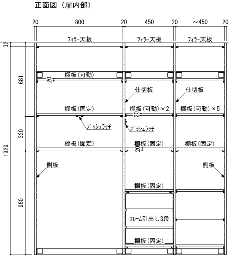
正面図（扉内部）
