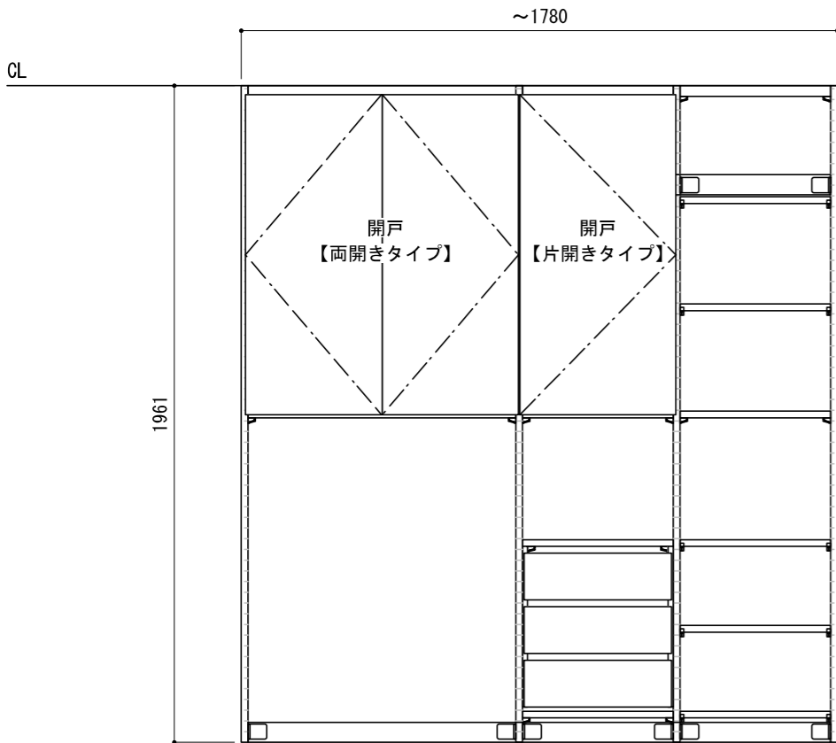
正面図（外観）
