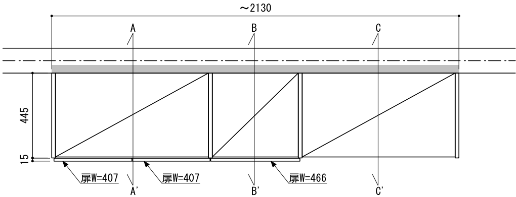
正面図（外観）
