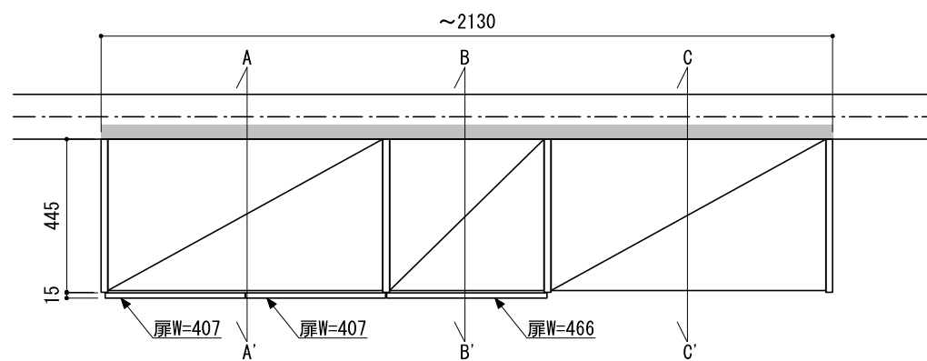
正面図（外觀）
