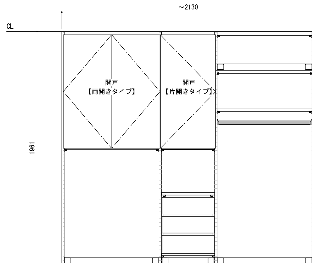
正面図（外觀）
