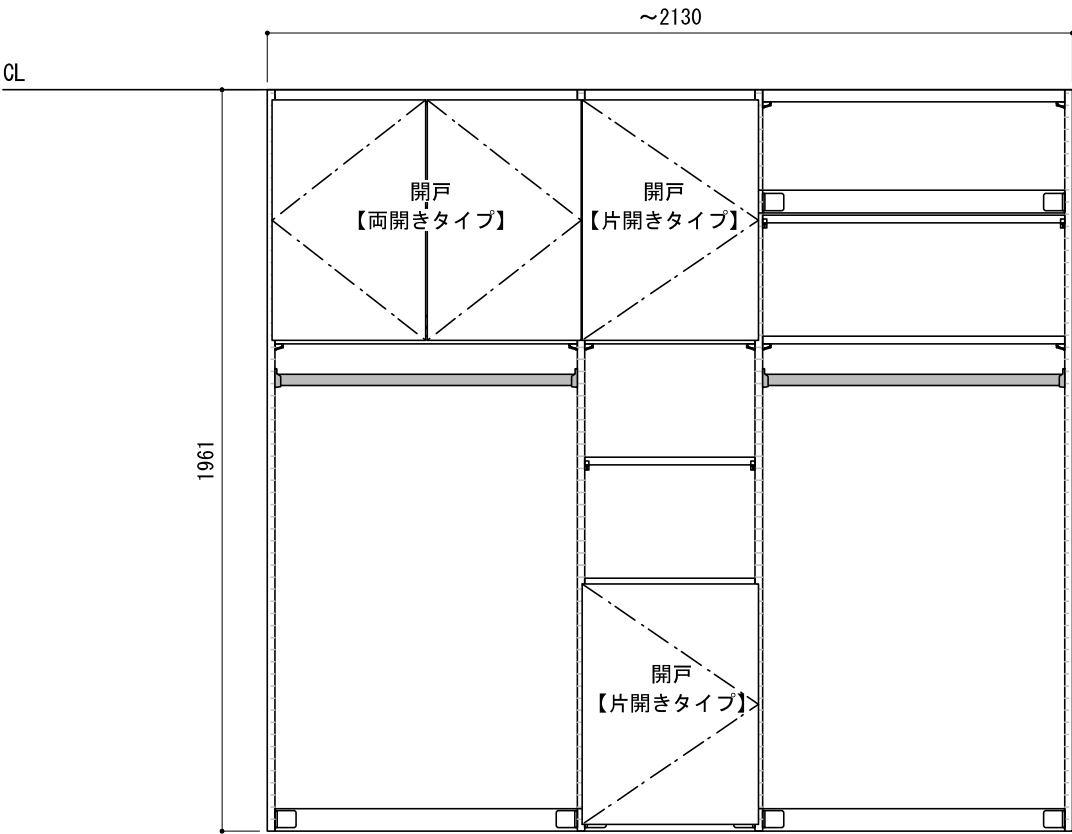
正面図（外観）
