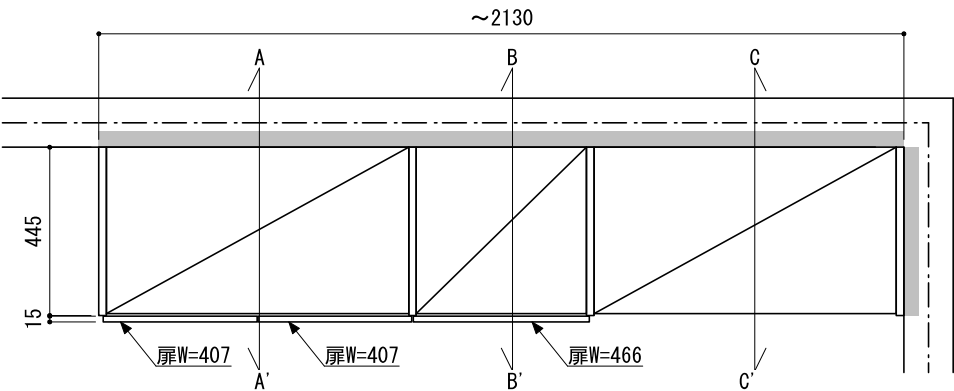
正面図（外観）
