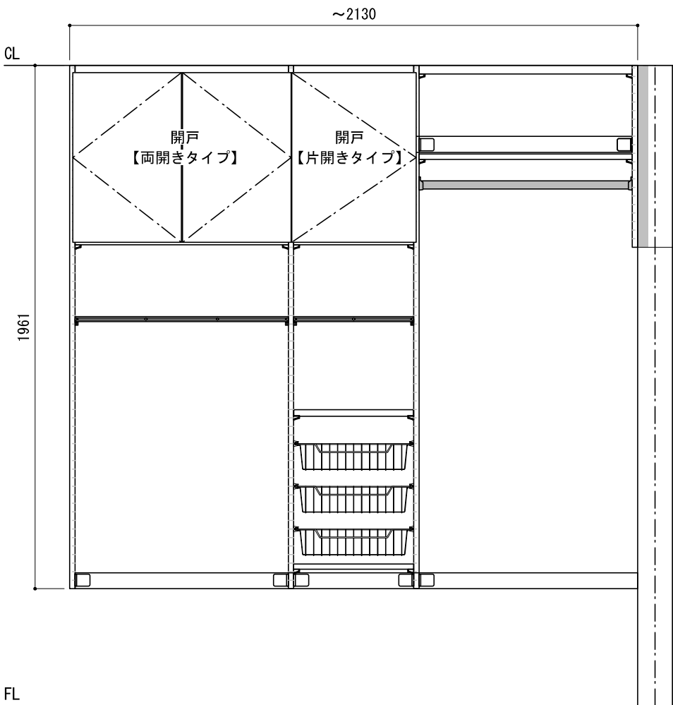
正面図（外観）
