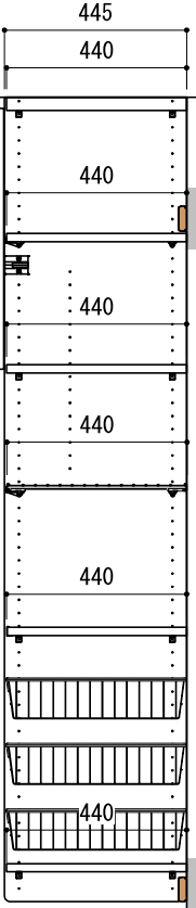
B-B' 断面
