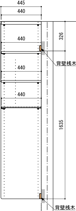
A-A' 断面
