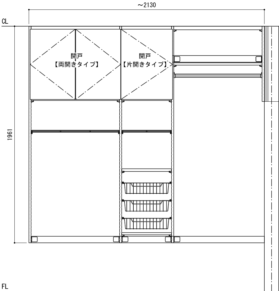
正面図（外観）
