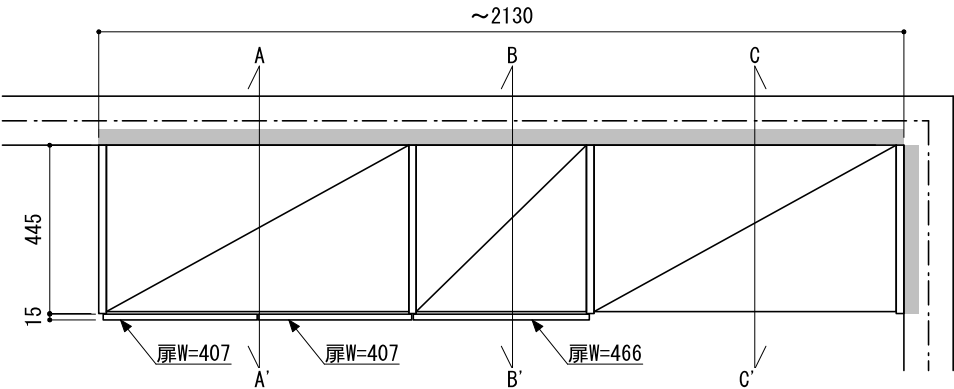
正面図（外観）
