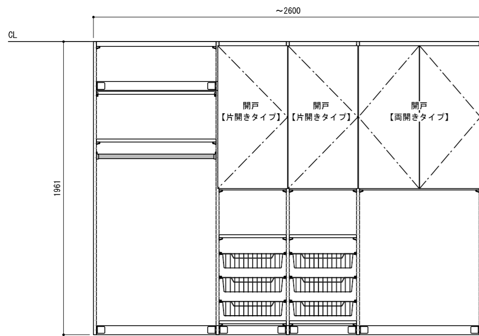
正面図（外観）
