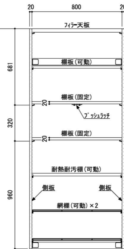
正面図（扉内部）
