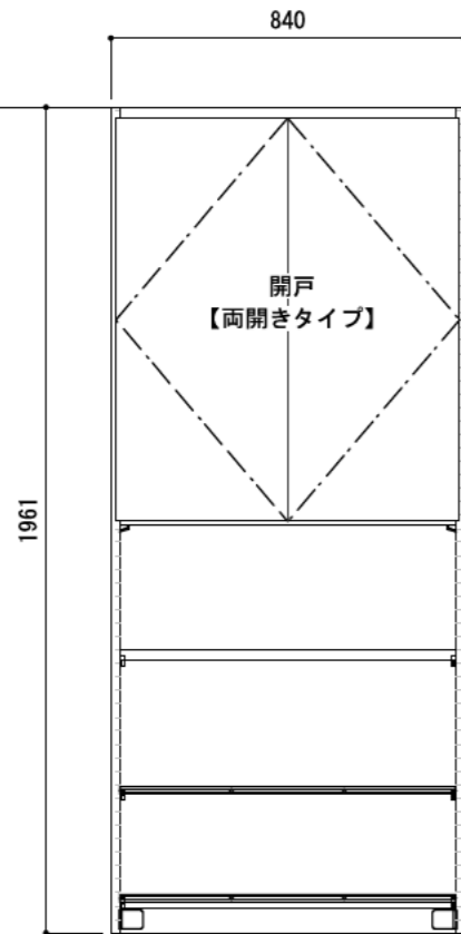
正面図（外観）
