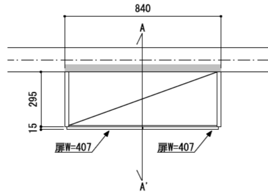
正面図（外観）
