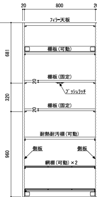
正面図（扉内部）
