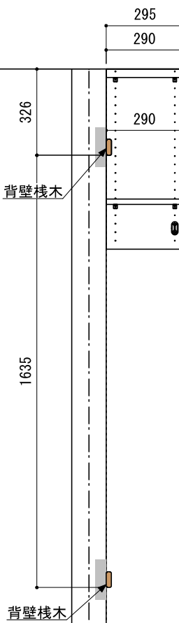
B-B' 断面
