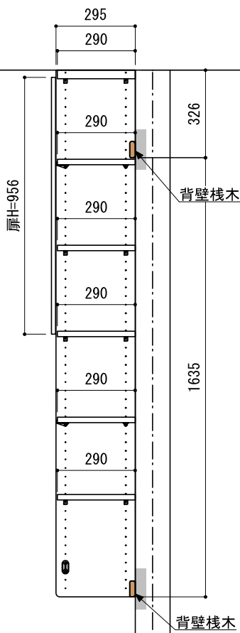
A-A' 断面
