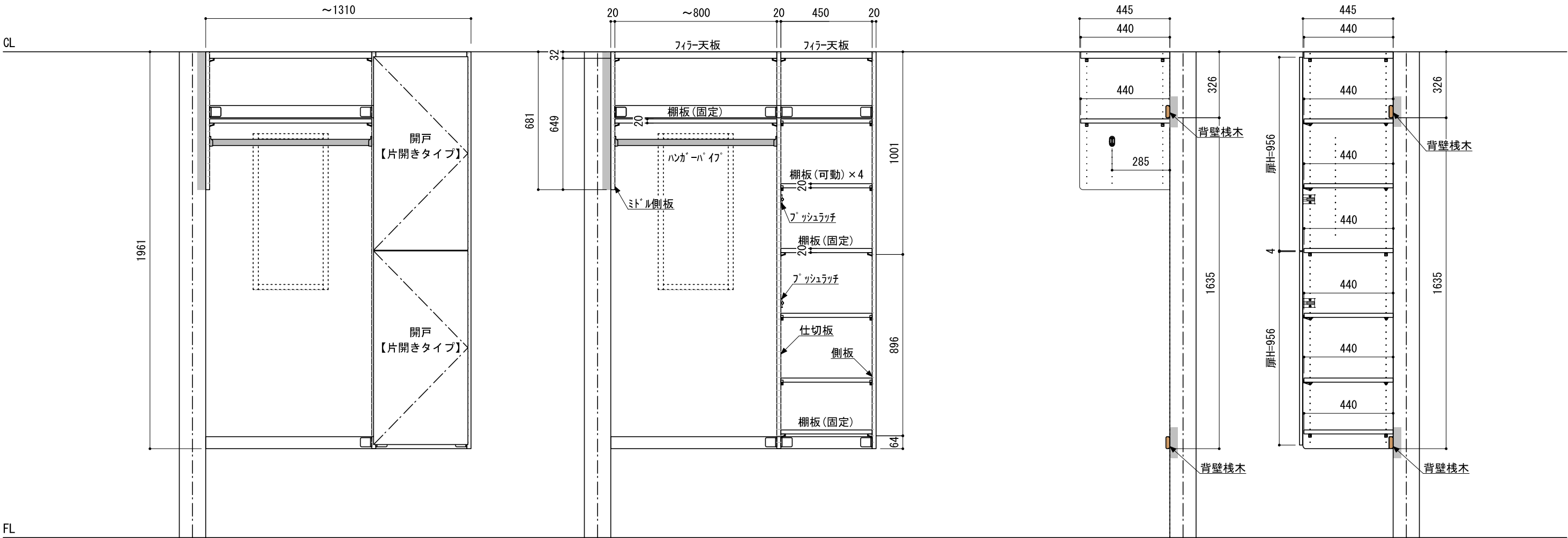
正面図（外観）
