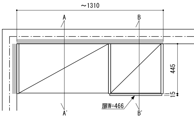
正面図（外観）
