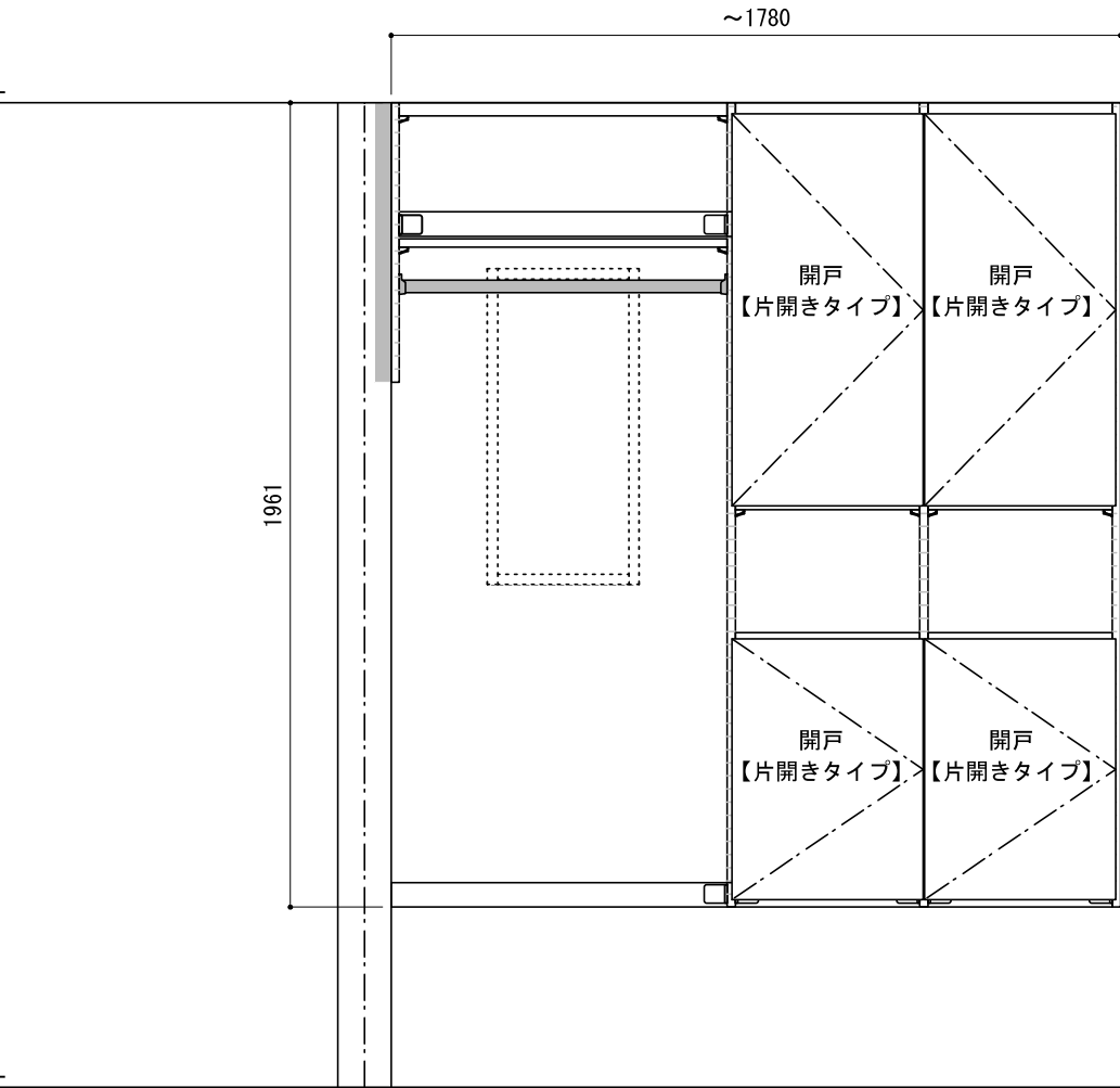
正面図（外観）
