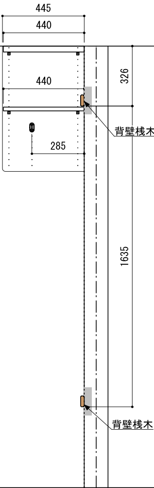
A-A' 断面
