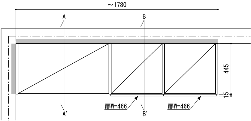
正面図（外観）
