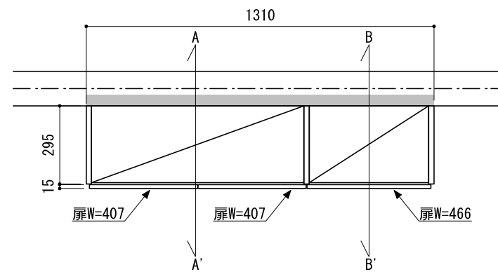
正面図（外観）
