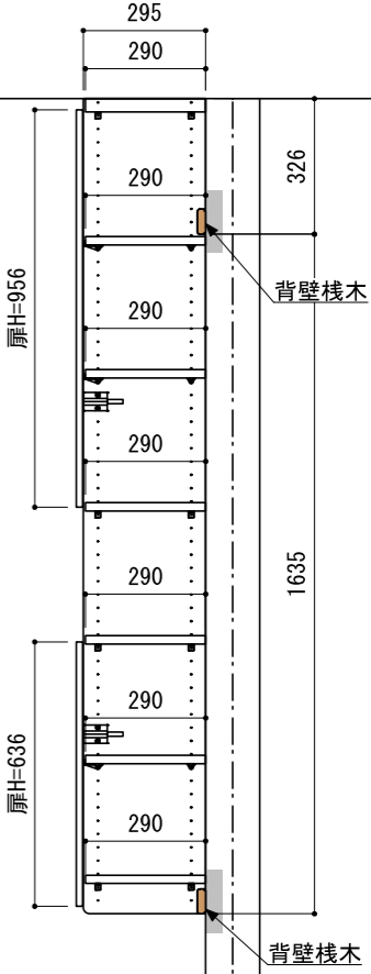
B-B' 断面
