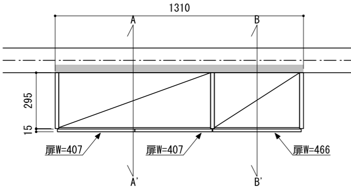
正面図（外観）
