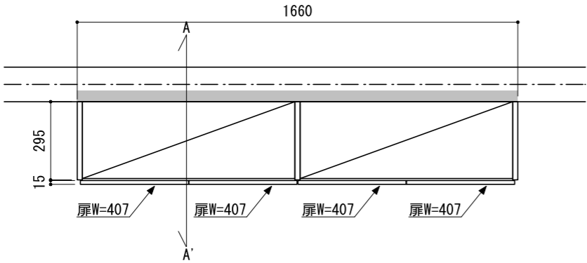
正面図（外観）
