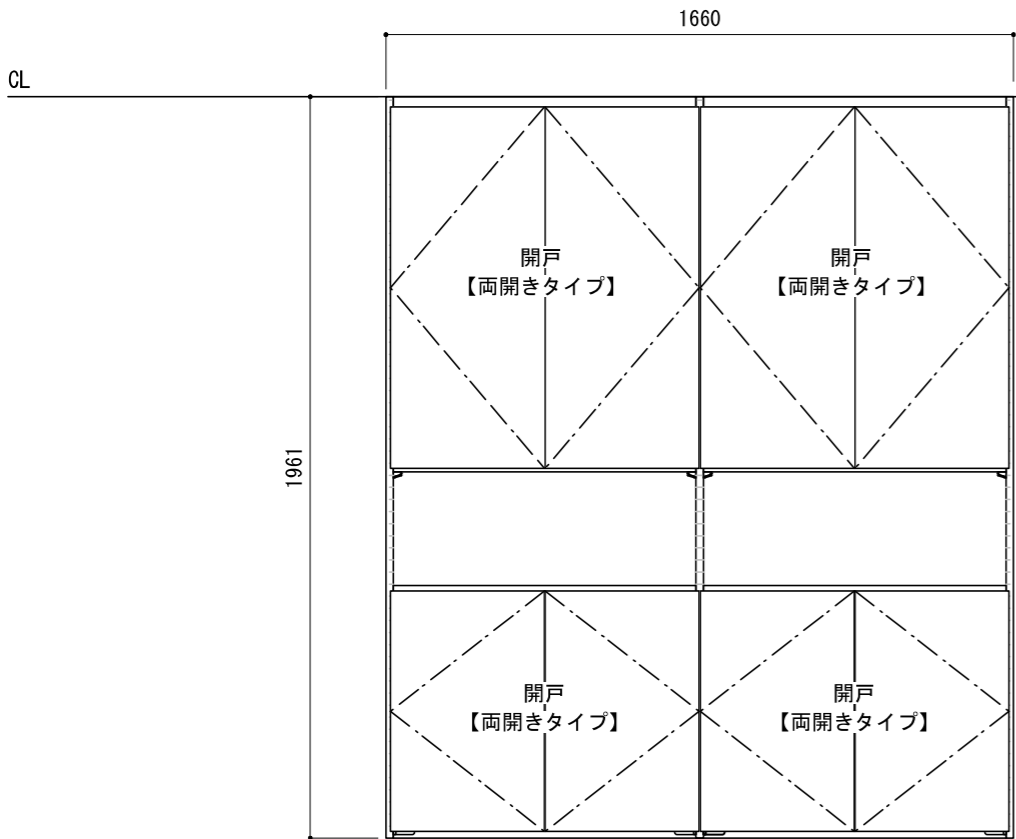
正面図（外観）
