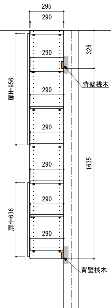
A-A' 断面
