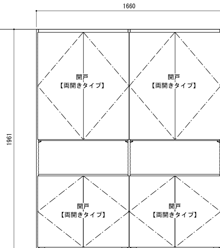
正面図（外観）
