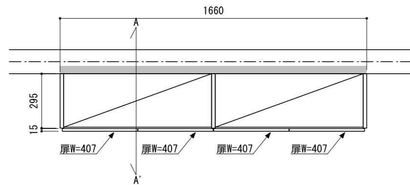
正面図（外観）
