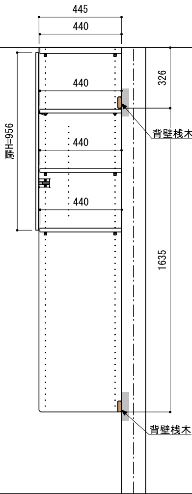
A-A' 断面
