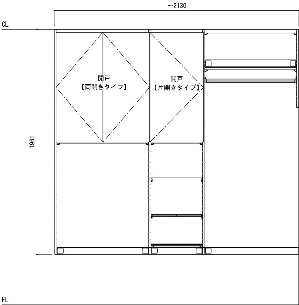
正面図（外観）
