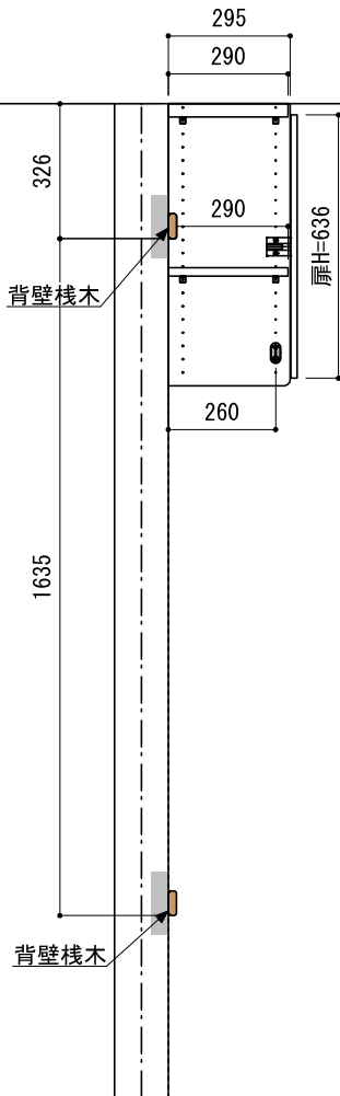
B-B' 断面
