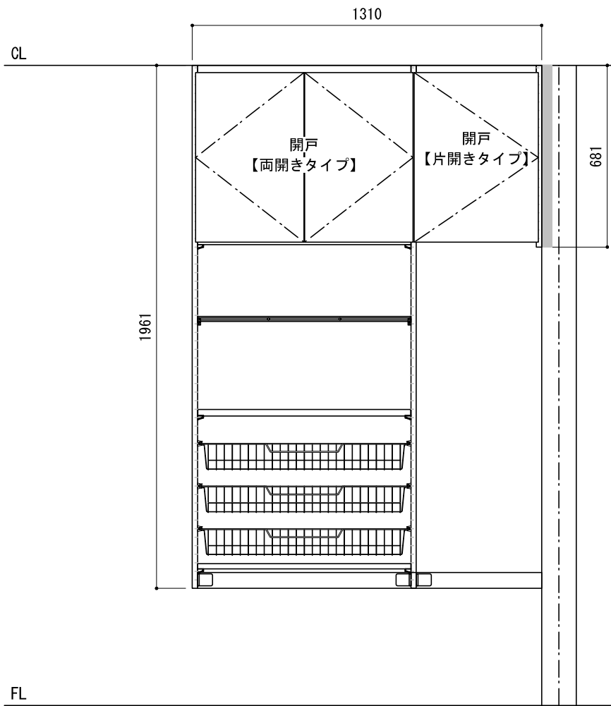
正面図（外観）
