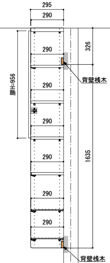
A-A' 断面
