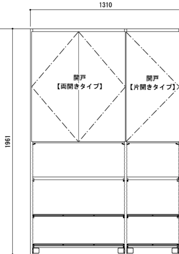
正面図（外観）
