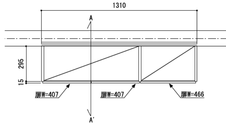
正面図（外観）
