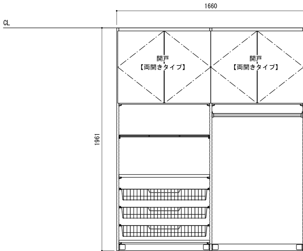
正面図（外観）
