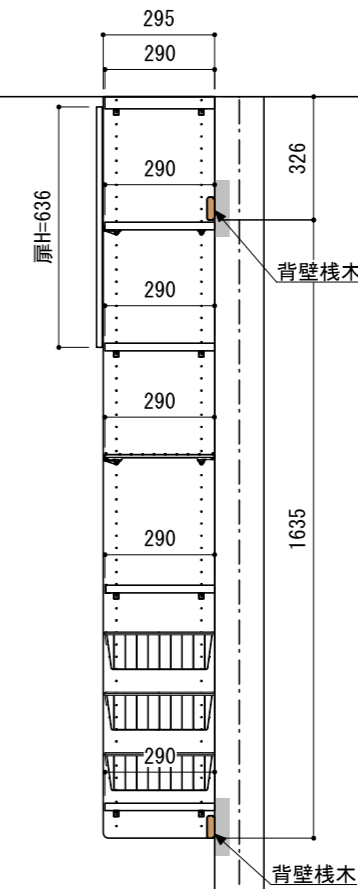
A-A' 断面
