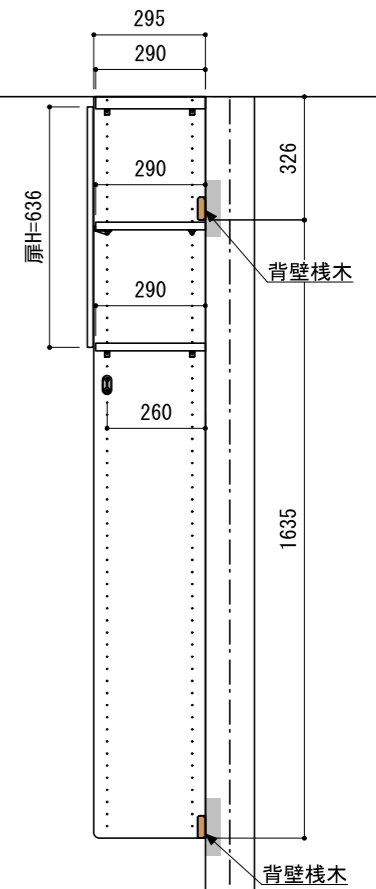
B-B' 断面
